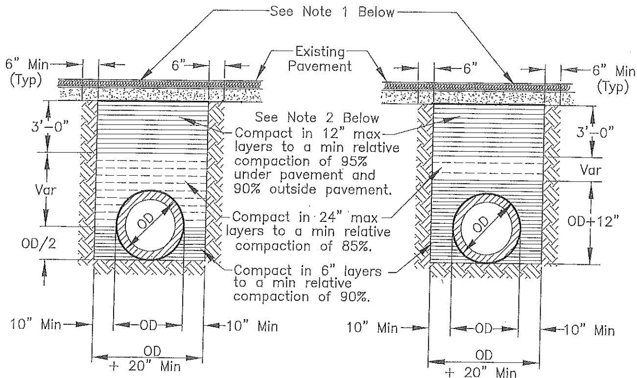
RIGID CONDUIT
